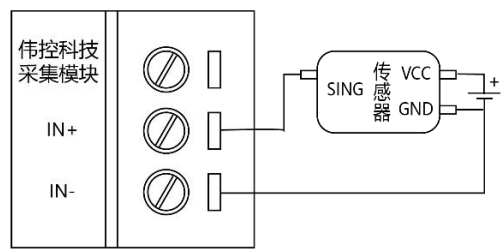
三线制传感器接法
