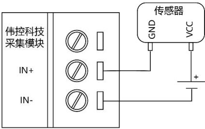
两线制传感器接法
