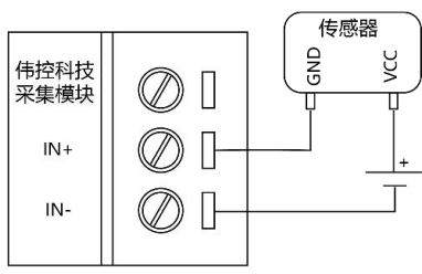
两线制传感器接法
