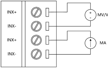
电压/电流可同时输入
