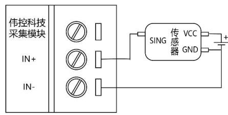
三线制传感器接法
