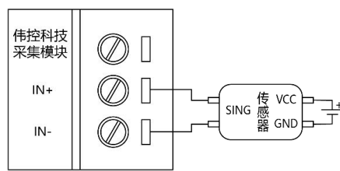
四线制传感器接法
