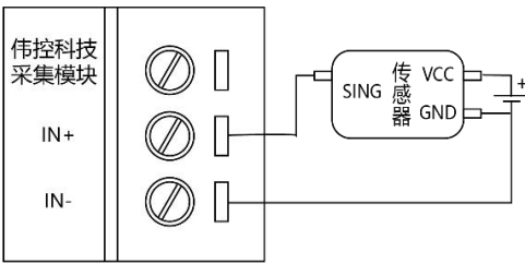
三线制传感器接法
