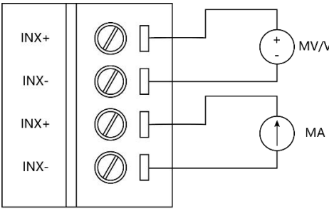
电压/电流可同时输入
